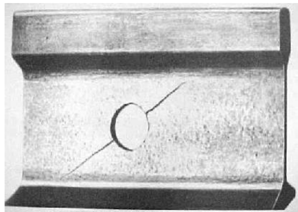
FIG. 45 : 135 OR 235 - WEB , CRACKS AT HOLE
